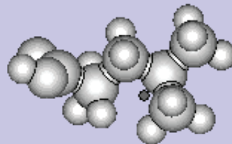
leucine.stl
