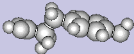
tyrosine.stl
