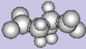
aspartate.stl
