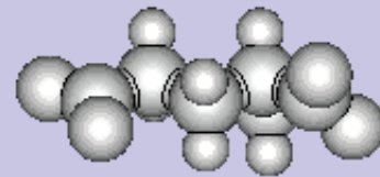
gluatamine.stl
