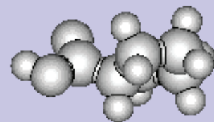
proline.stl
