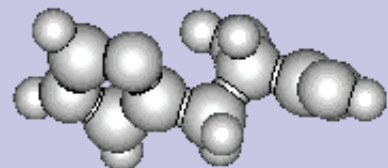
histadine.stl
