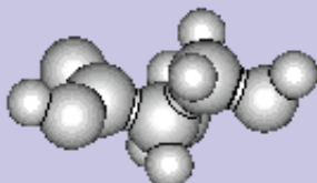
serine.stl
