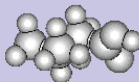
valine.stl
