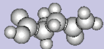
asparagine.stl
